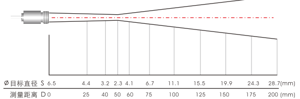
Optics CTLT CF, D:S=22:1 (远距离=6:1)
