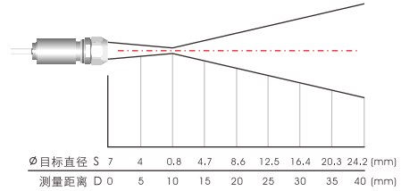
15:1带CF透镜(远距离=1.5:1)
